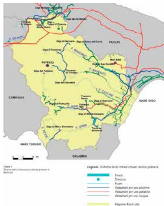
Figura 23. Schema idrico regionale
